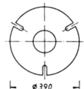
Erdstück E4 für Kandelaber Nr. 620, 640
