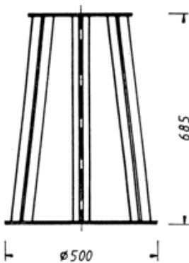
Erdkorb E1 für Kandelaber Nr. 600, 610, 630, 650, 660 und 670
