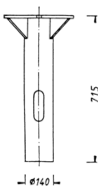
Erdstück E3 für Kandelaber Nr. 600, 610, 630, 650, 660 und 670
