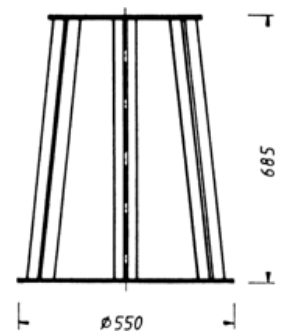
Erdkorb E2 für Kandelaber Nr. 620, 640
