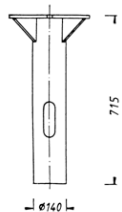
Erdstück E4 für Kandelaber Nr. 620, 640
